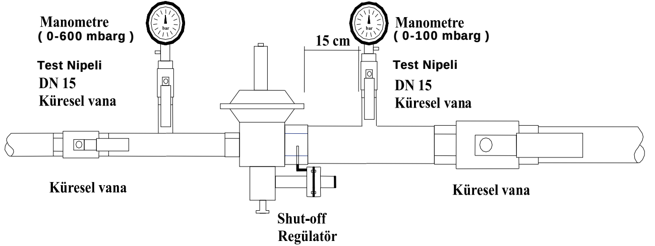
Şekil 13 Shut-Off Regülatör
