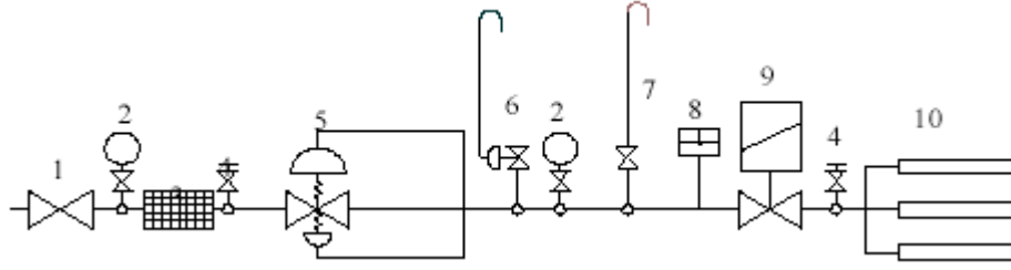
Şekil 32 Atmosferik brülör doğa! gaz kontrol hattı ekipmanları
