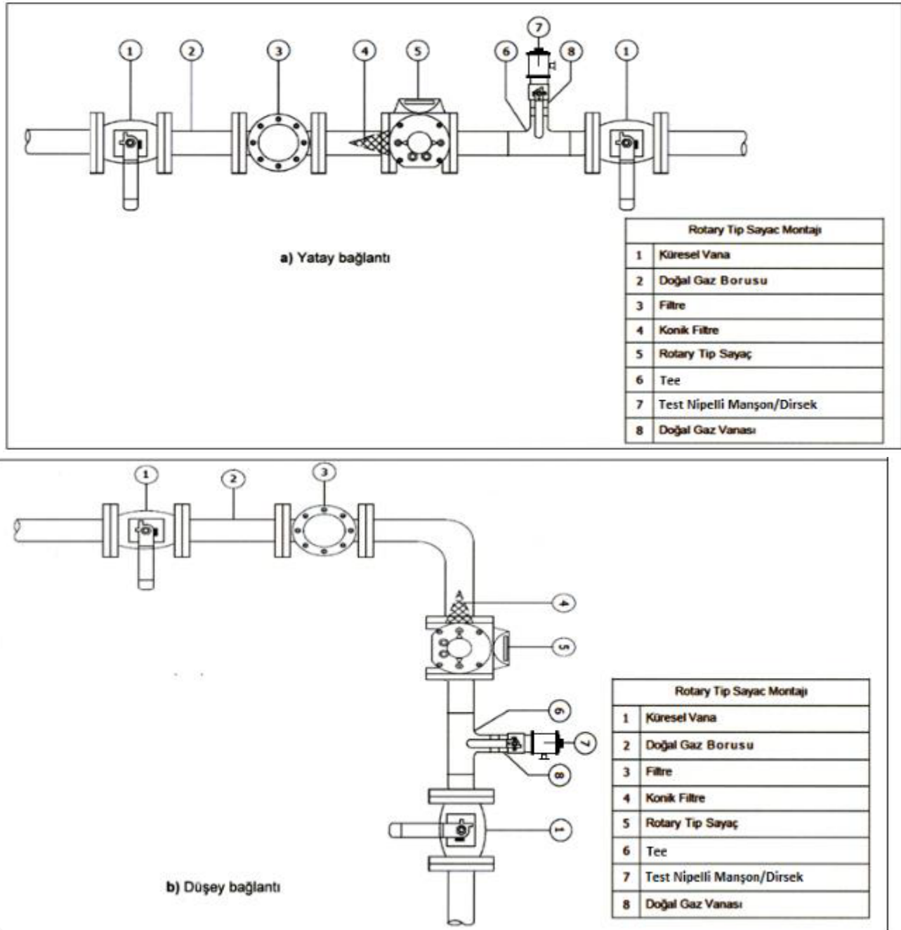
Şekil 16 — Rotary sayaçlara ait bağlantı detayı
