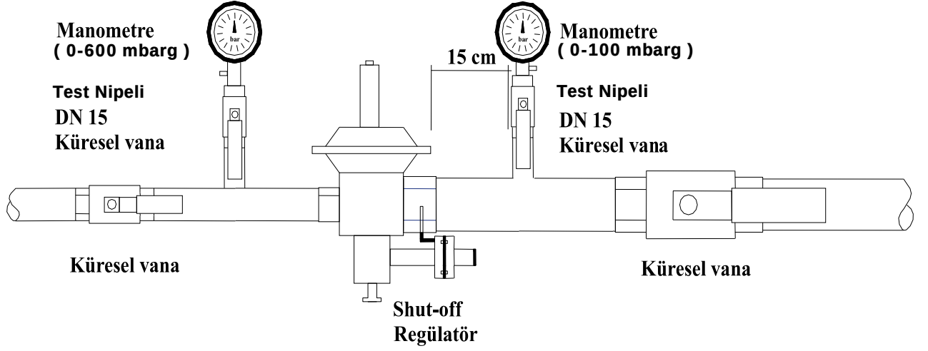
Şekil 13 Shut-Off Regülatör
